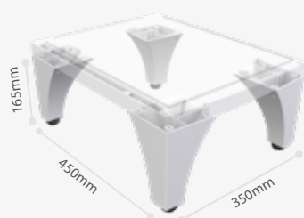
NK 1512 Pé elevado em ABS
