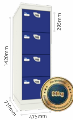
NK 1723 (Armário Gaveteiro)
